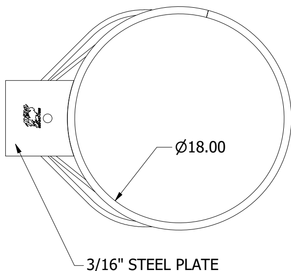
TOP
